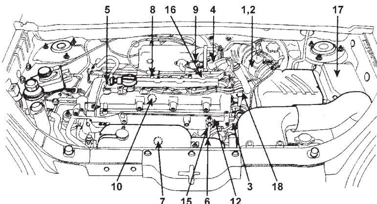
<Двигатель 2.7L>
