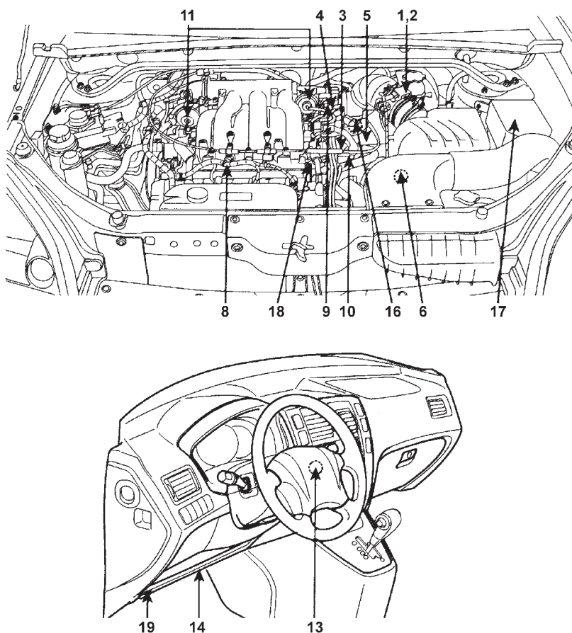
<Двигатель 2.7L>
