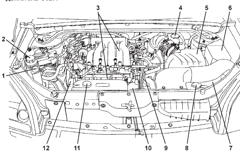
<Двигатель G6BA>
