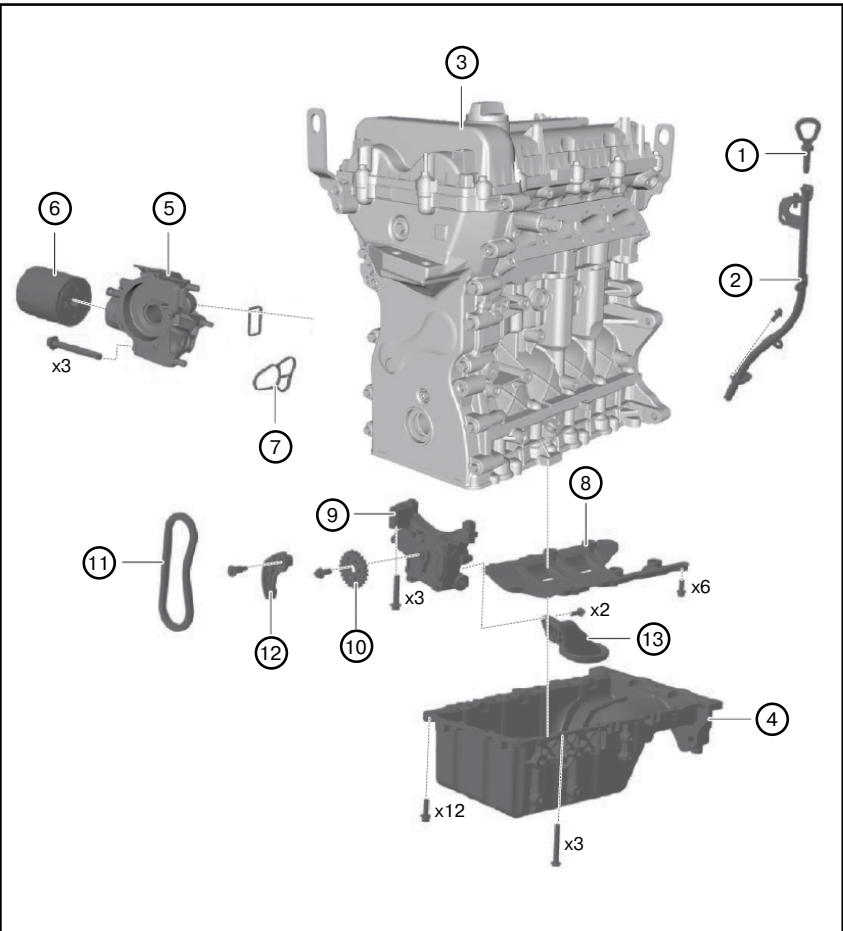
Двигатель 1,5 л 1. Маслоизмерительный щуп. 2. Трубка маслоизмерительного щупа. 3. Крышка маслосаливной горловины. 4. Масляный поддон. 5. Модуль масляного фильтра. 6. Масляный фильтр. 7. Уплотнительное кольцо (заменять новым после каждого снятия). 8. Маслоотражатель. 9. Масляный насос. 10. Звездочка привода масляного насоса. 11. Цепь привода масляного насоса. 12. Подвижная направляющая планка цепи привода масляного насоса. 13. Маслоприемник.
