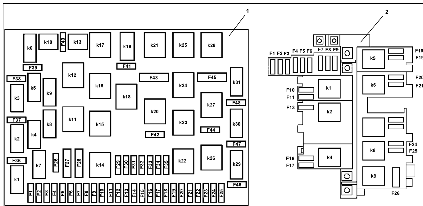
1 - монтажный блок в подкапотном пространстве, 2 - монтажный блок в салоне.
