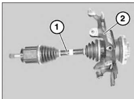
Рис. 13.8. Приводной вал
