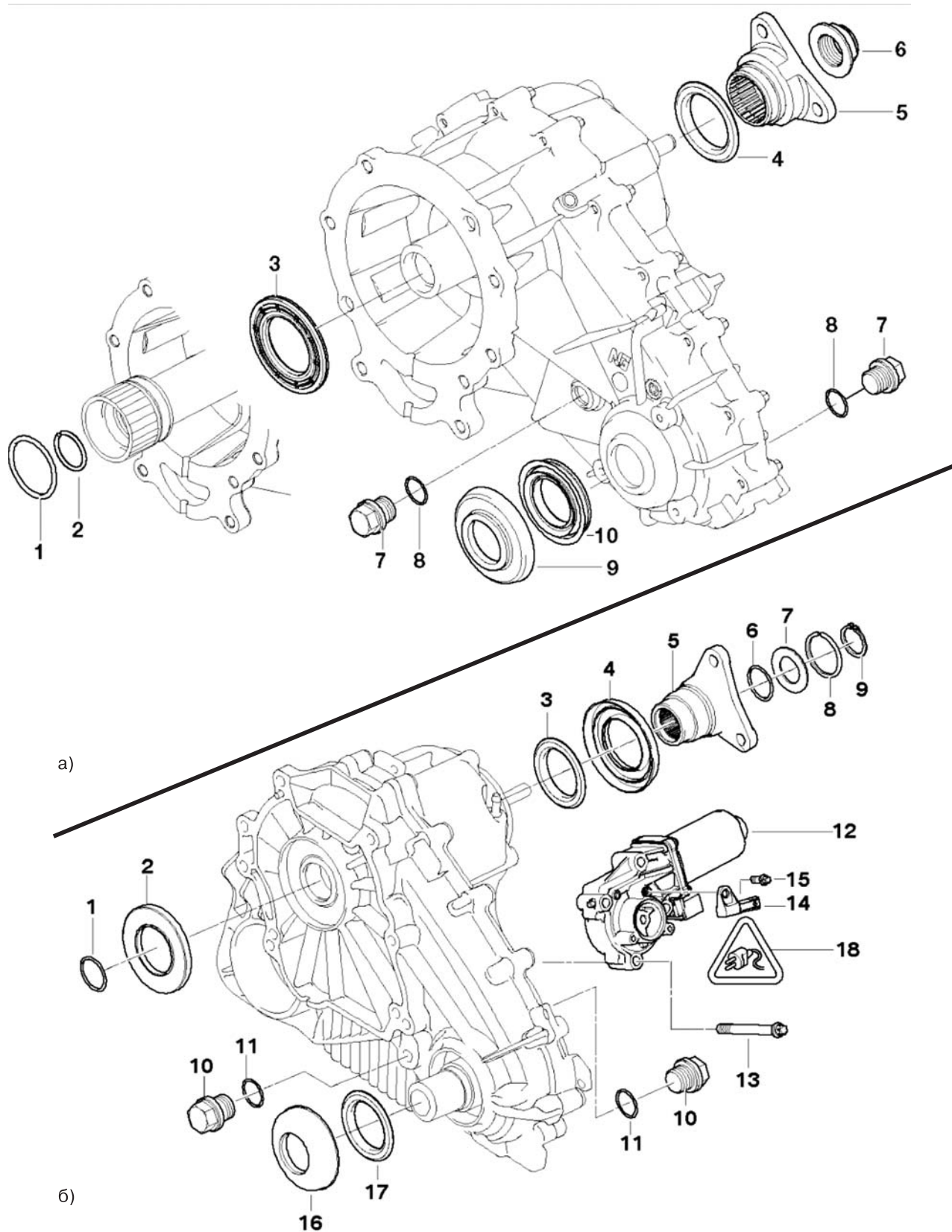
Рис. 10.1. Раздаточная коробка:
