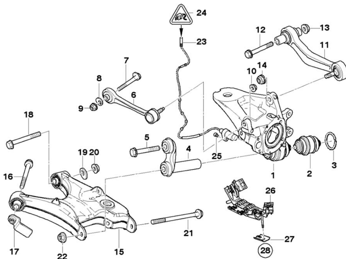
Рис. 14.3. Подвеска колеса:
