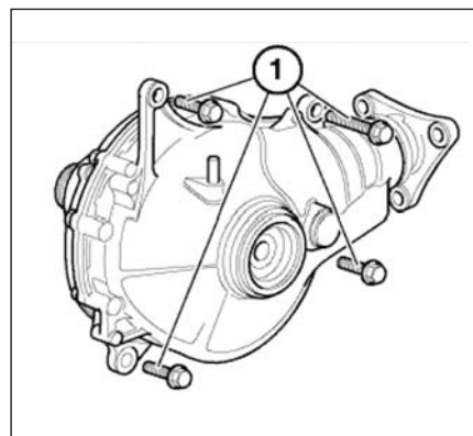
Рис. 13.10. Редуктор переднего моста
