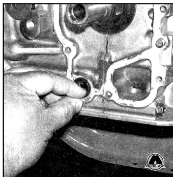
15.21 Установите новое уплотнительное кольцо между корпусом насоса и блоком цилиндров
