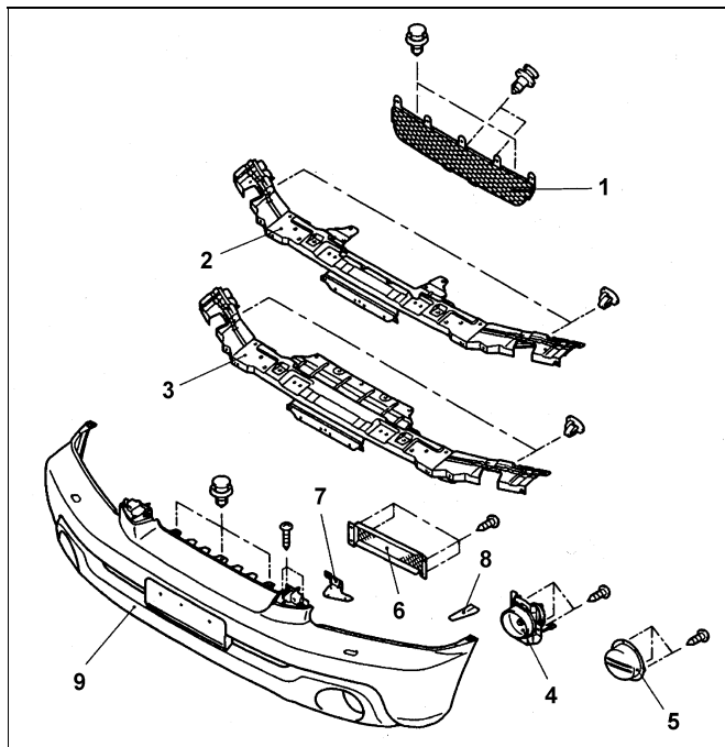
Разборка переднего бампера. 1 - декоративная решетка переднего бампера (модели с двигателем 4G94), 2 - элемент жесткости переднего бампера (модели с двигателем 4G94), 3 - элемент жесткости переднего бампера (модели с двигателем 4G93), 4 - передняя противотуманная фара, 5 - заглушка (модели без передних противотуманных фар), 6 - декоративная сетка переднего бампера, 7 - передний кронштейн крепления накладки бампера, 8 - боковой кронштейн крепления накладки бампера, 9 - накладка переднего бампера.
