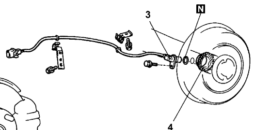
<Заднее колесо>
