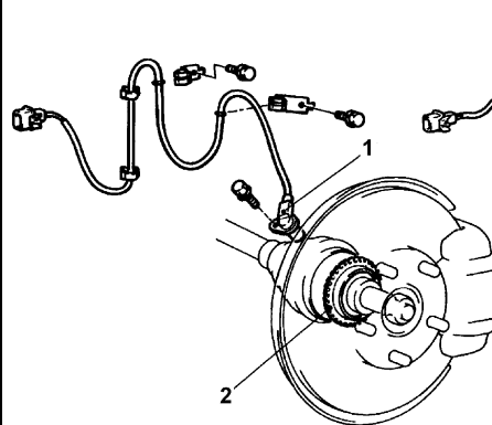
<Переднее колесо>
