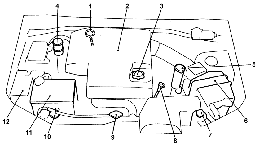
<Двигатель 4G93-MPI>
