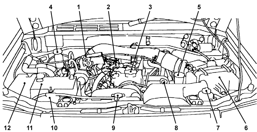
<Двигатель 4G93-MPI>
