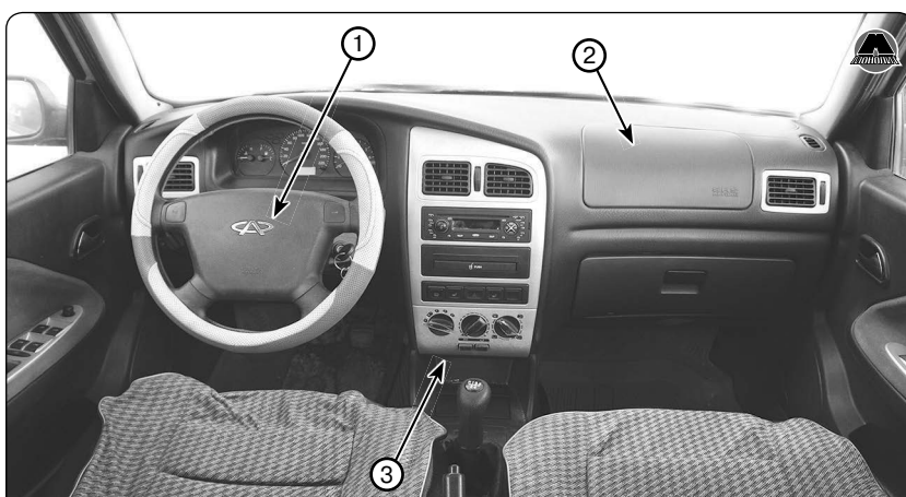
1. Модуль подушки безопасности водителя. 2. Модуль подушки безопасности пассажира. 3. Место расположения блока управления дополнительной пассивной безопасности.
