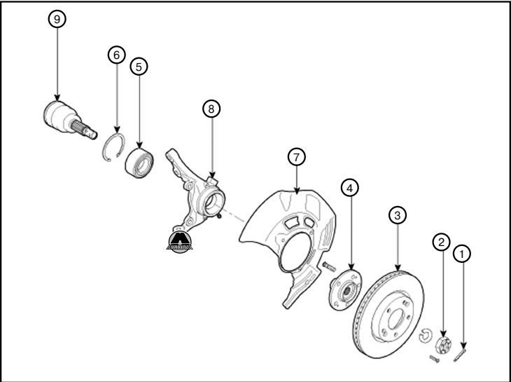
1. Шплинт. 2. Корончатая гайка. 3. Тормозной диск. 4. Ступица. 5. Колесный подшипник. 6. Стопорное кольцо. 7. Пылезащитный чехол. 8. Поворотный кулак. 9. Приводной вал.
