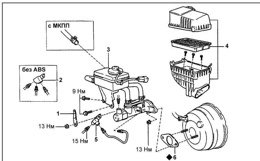
Снятие главного тормозного цилиндра (Picnic). 1 - кронштейн, 2 - тройник, 3 - главный тормозной цилиндр, 4 - воздушный фильтр в сборе, 5 - переходник, 6 - прокладка.
