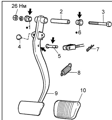
Педали тормоза. 1 - седло, 2 - втулка, 3 - болт, 4 - упор, 5 - ось вилки, 6 - седло, 7 - шплинт, 8 - возвратная пружина, 9 - педаль тормоза, 10 - накладка.
