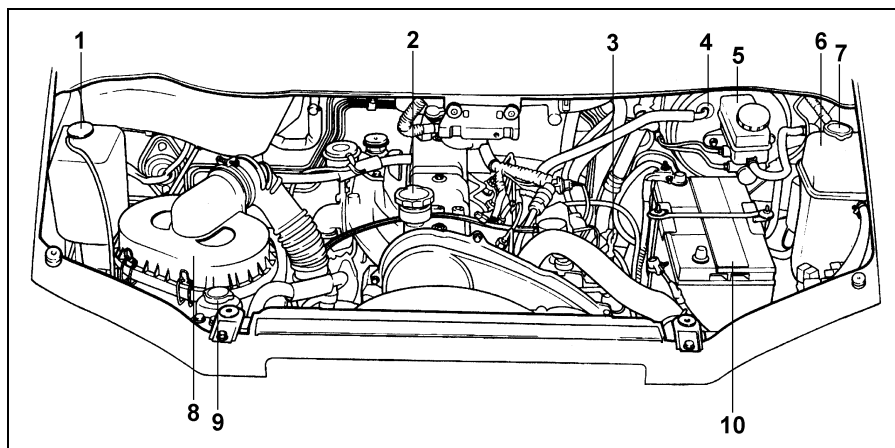
Расположение компонентов в моторном отсеке (модели до 2004 г., один из вариантов). 1 - бачок омывателя, 2 - крышка маслозаливной горловины двигателя, 3 - щуп уровня моторного масла, 4 - вакуумный усилитель тормозов, 5 - бачок тормозной системы и гидропривода выключения сцепления, 6 - расширительный бачок системы охлаждения двигателя, 7 - крышка расширительного бачка, 8 - воздушный фильтр, 9 - бачок гидроусилителя рулевого управления, 10 - аккумуляторная батарея.
