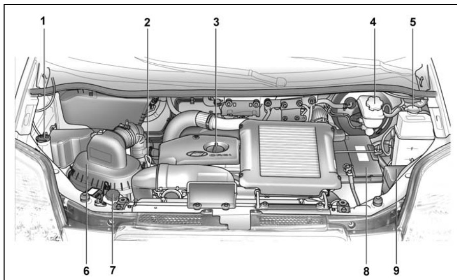
Расположение компонентов в моторном отсеке (D4CB (2,5 л, CRDi)). 1 - бачок омывателя, 2 - щуп уровня моторного масла, 3 - крышка маслозаливной горловины двигателя, 4 - бачок тормозной системы, 5 - расширительный бачок системы охлаждения двигателя, 6 - воздушный фильтр, 7 - бачок гидроусилителя рулевого управления, 8 - аккумуляторная батарея, 9 - блок реле и предохранителей в моторном отсеке.
