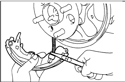
Задние барабанные тормоза (модели 2WD).
