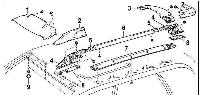
Направляющая для крепления багажника (тип 2). 1 - панель дефлектора, 2 - декоративная крышка багажника, 3 - спойлер задней двери, 4 - опорный кронштейн, 5 - уплотнение, 6 - направляющая для крепления багажника, 7 - декоративная накладка крыши, 8 - прокладка, 9 - заглушка.
