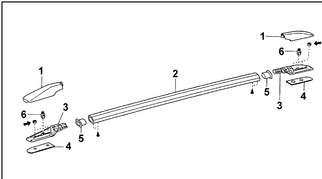
Направляющая для крепления багажника (тип 1). 1 - декоративная крышка опорного кронштейна, 2 - направляющая для крепления багажника, 3 - опорный кронштейн, 4 - прокладка, 5 - уплотнение, 6 - пистон.
