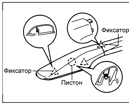
Передняя декоративная крышка опорного кронштейна.
