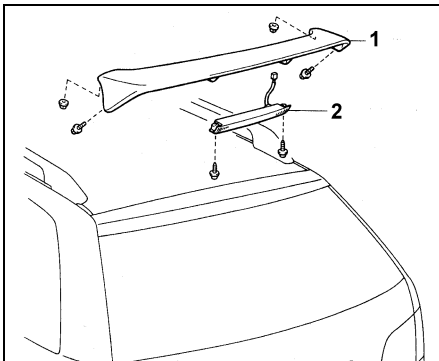
Тип 1. 1 - спойлер задней двери, 2 - дополнительный стоп-сигнал.
