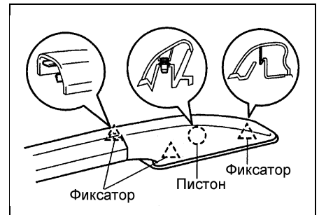
Задняя декоративная крышка опорного кронштейна.
