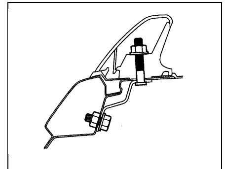
Тип 2. 1, 2 - уплотнитель спойлера задней двери, 3 - шайба, 4 - спойлер задней двери, 5 - отделка задней двери.
