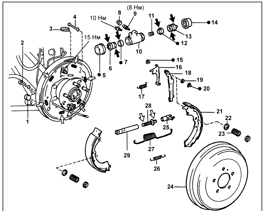
Задние барабанные тормоза (модели 4WD).
