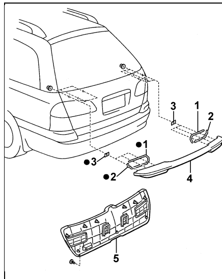
Тип 2. 1, 2 - уплотнитель спойлера задней двери, 3 - шайба, 4 - спойлер задней двери, 5 - отделка задней двери.
