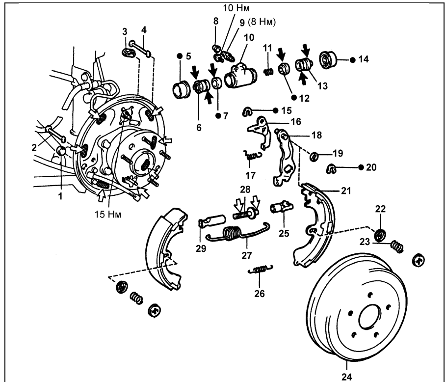
Задние барабанные тормоза (модели 2WD).
