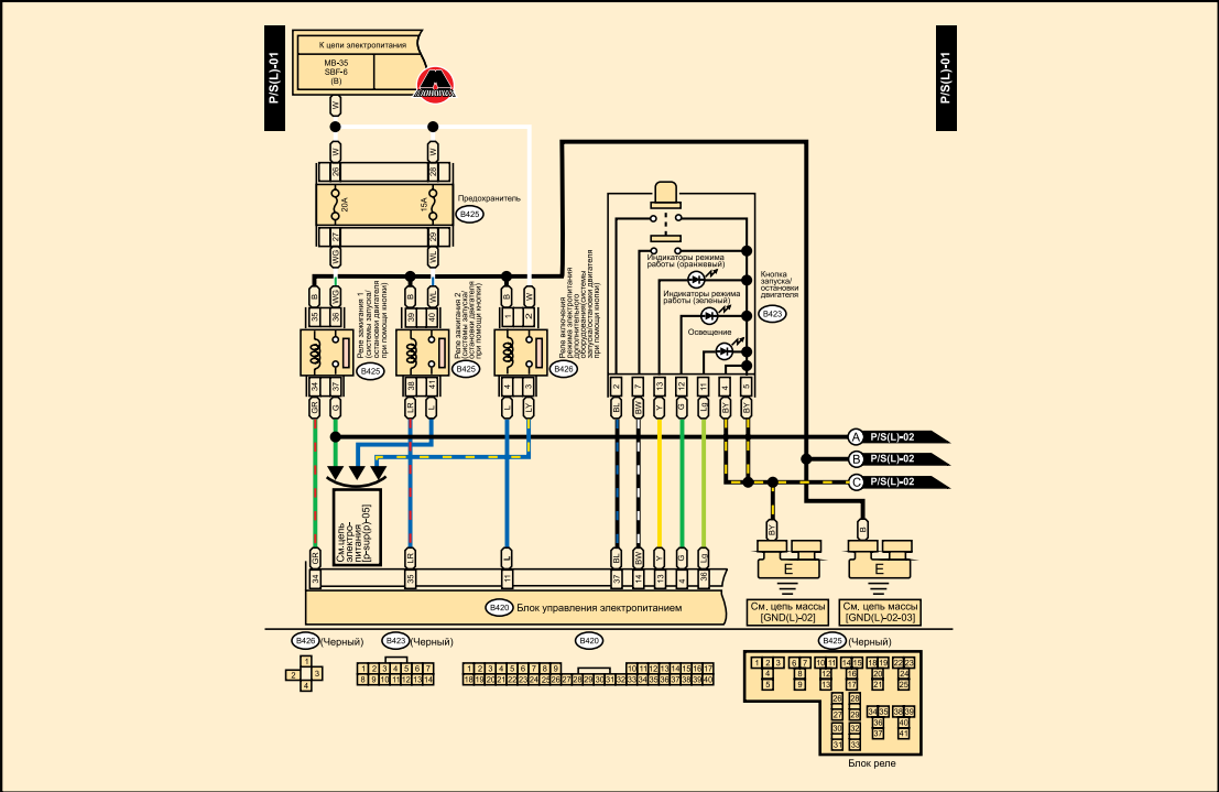
ЭЛЕКТРОСХЕМА СИСТЕМЫ ЗАПУСКА/ОСТАНОВКИ ДВИГАТЕЛЯ ПРИ ПОМОЩИ КНОПКИ (2)
