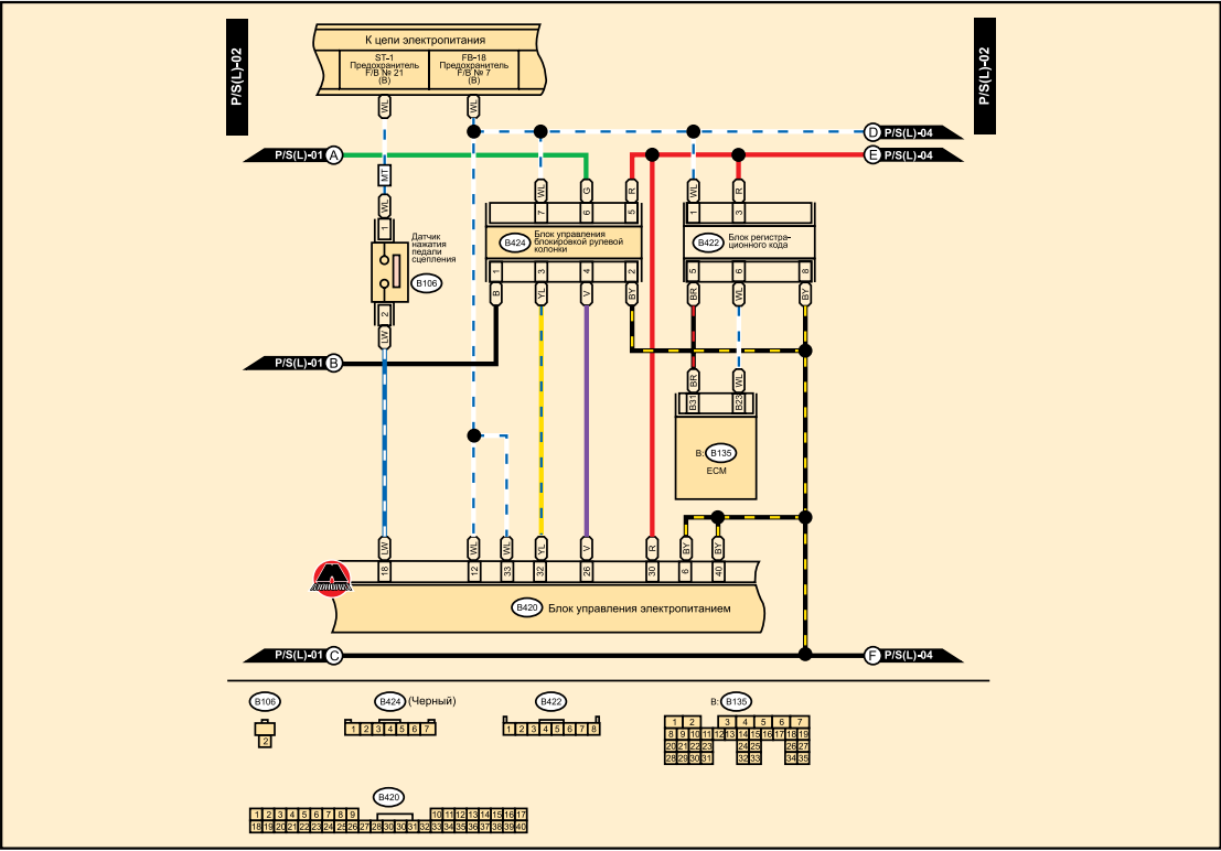
ЭЛЕКТРОСХЕМА СИСТЕМЫ ЗАПУСКА/ОСТАНОВКИ ДВИГАТЕЛЯ ПРИ ПОМОЩИ КНОПКИ (2)
