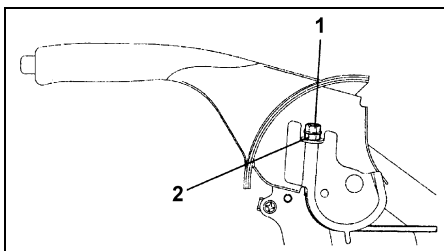
1 - контргайка, 2 - регулировочная гайка.
