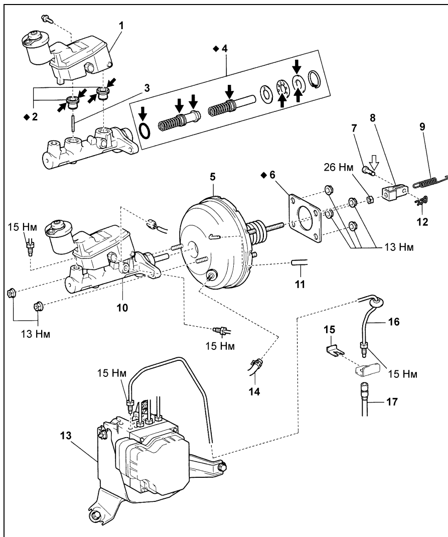
Главный тормозной цилиндр (с VSC). 1 - бачок, 2 - резиновые втулки, 3 - штифт, 4 - элементы главного тормозного цилиндра, 5 - вакуумный усилитель тормозов, 6 - прокладка, 7 - ось вилки, 8 - вилка, 9 - пружина, 10 - главный тормозной цилиндр в сборе, 11 - шланг, 12 - шплинт, 13 - модулятор давления, 14 - вакуумный шланг №1, 15 - фиксатор, 16 - трубка №4 передних тормозов, 17 - тормозной шланг.
