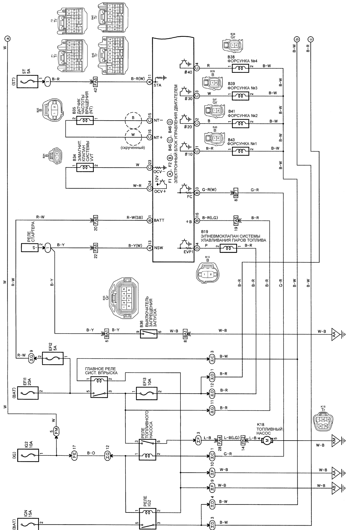
СИСТЕМА УПРАВЛЕНИЯ ДВИГАТЕЛЕМ И АКПП (модели с двигателем 1ZZ-FE)
