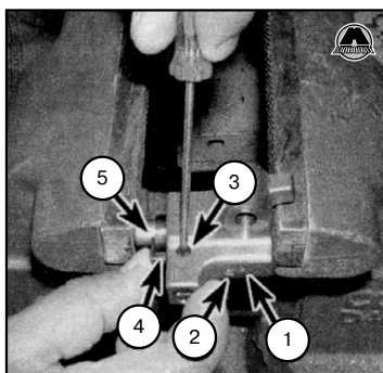
7.27 Во время фиксации натяжителей вторичных цепей привода учитывайте метки на боковой стороне натяжителей, так как натяжители не взаимозаменяемые. 1. Установите стопорный штифт 2. Идентификационная метка 3. Храповая собачка 4. Храповой механизм 5. Поршень натяжителя
