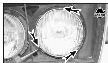
1. Регулировочный винт. 2. Стрелки, указывающие направление наклона отражателя.
