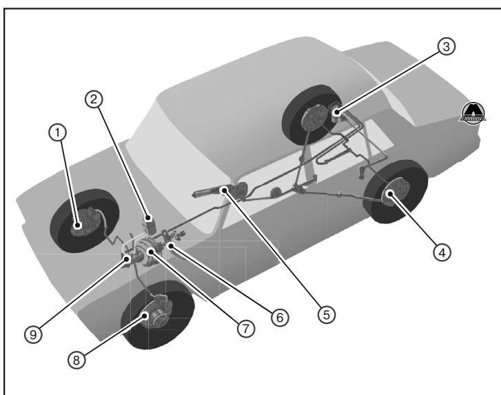
1. Тормозной щит переднего тормоза, 2. Расширительный бачок для тормозной жидкости, 3. Регулятор давления задних тормозов, 4. Тормозной барабан, 5. Рычаг стояночного тормоза, 6. Педаль тормоза, 7. Вакуумный усилитель, 8. Тормозной диск, 9. Главный тормозной цилиндр.
