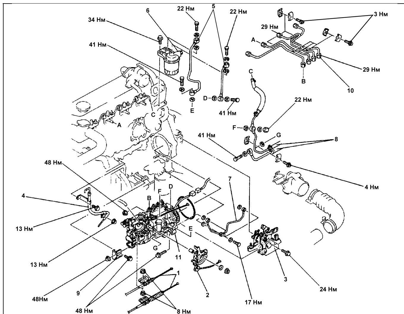
Регулирующая точка Положение рейки ТНВД, мм Частота вращения вала ТНВД, об/мин Число циклов Объём впрыска, см 3 /1000 циклов Погрешность (%) Управление Примечание A 11,3 900 1000 69,6 - 72,8 ±2,5 Рейка Основной H около 9,5 290 1000 6,7 - 9,3 ±14,0 Рейка - A R1 11,2 900 1000 70,2 - 72,2 - Рычаг Избыточное давление около 110 мм рт. ст. B R1 - 0,25 550 1000 (49,7) - Рычаг Избыточное давление около 110 мм рт. ст. C 10,2 550 1000 (29,7) - Рычаг - D R1 - 0,2 1500 1000 78,0 - Рычаг Избыточное давление около 110 мм рт. ст. E - 150 1000 Около 90,0 - Рычаг -
