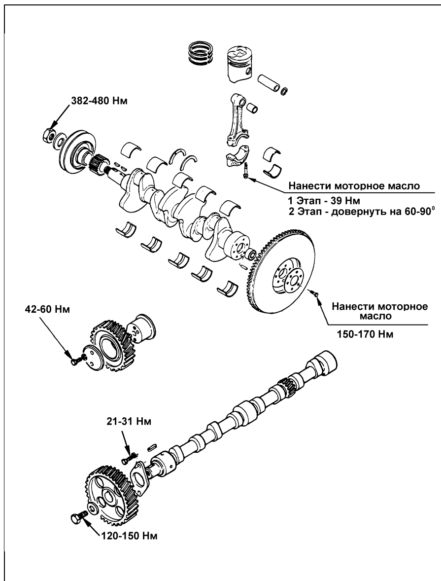
Коленчатый и распределительный вал (4BD1, 4BD1-T).
