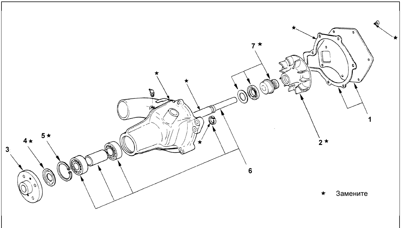
Разборка и сборка насоса охлаждающей жидкости. 1 - крышка корпуса, 2 - крыльчатка насоса, 3 - фланец, 4 - шайба, 5 - стопорное кольцо, 6 - вал в сборе, 7 - уплотнитель.
