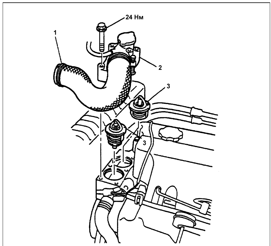
Снятие и установка термостата (4HF1, 4HG1). 1 - шланг, 2 - крышка корпуса термостата, 3 - термостат.
