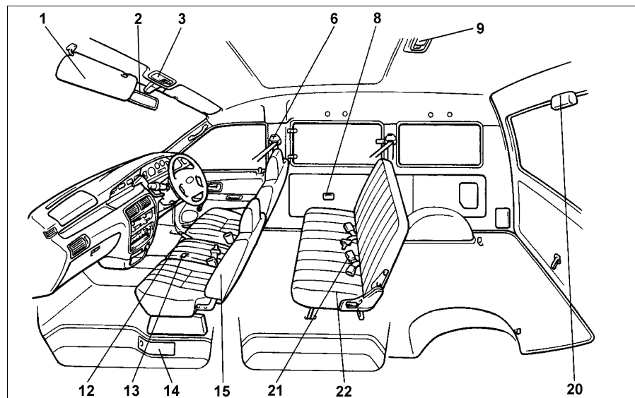
Расположение элементов в салоне (комплектация SW).
