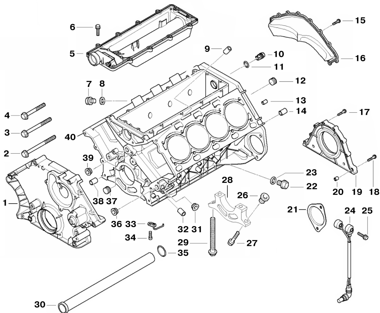
Рис. 4.2. Блок цилиндров:
