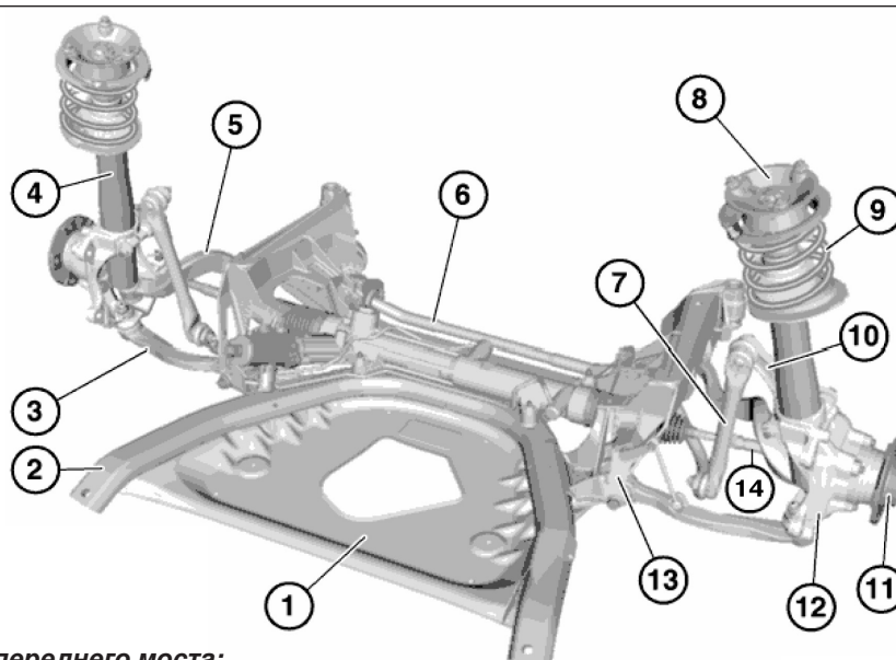
Рис. 12.1. Компоновка переднего моста:
