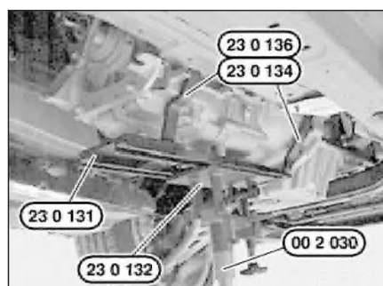
Рис. 7.8. Приспособление «23.0.130»
