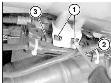
Рис. 7.7. Фиксаторы
