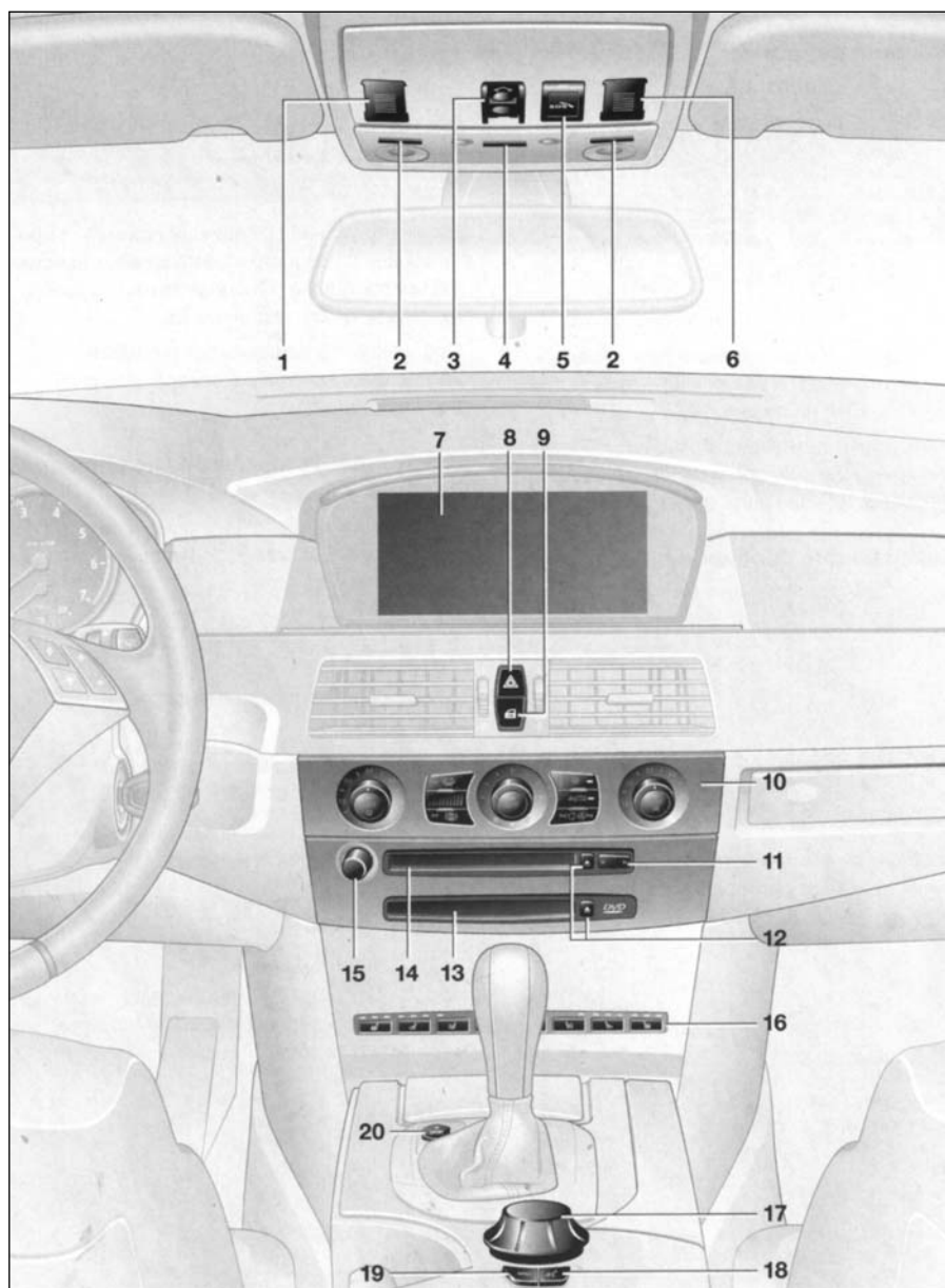
Рис. 1.9. Зона центральной консоли:
