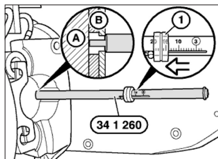
Рис. 11.5. Индикатор
