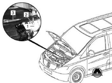
1. Расширительный бачок. 2. Контрольная пробка. 3. Нагнетательный насос.
