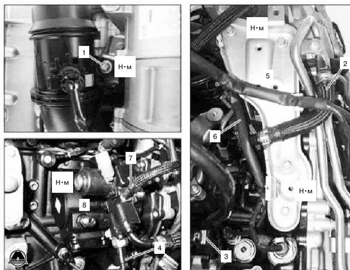
1. Болт. 2. Топливопровод. 3. Вакуумная магистраль. 4. Электрический разъем. 5. Кронштейн. 6. Электропроводка. 7. Возвратный топливопровод. 8. Топливный насос высокого давления.
