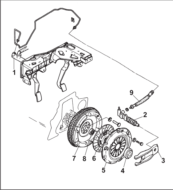
1 - Главный цилиндр, 2 - Рабочий цилиндр, 3 - Вилка выключения сцепления, 4 - Выжимной подшипник, 5 - Корзина сцепления, 6 - Диск сцепления, 7 - Маховик, 8 - Опорный подшипник вала КПП, 9 - Гибкий шланг.
