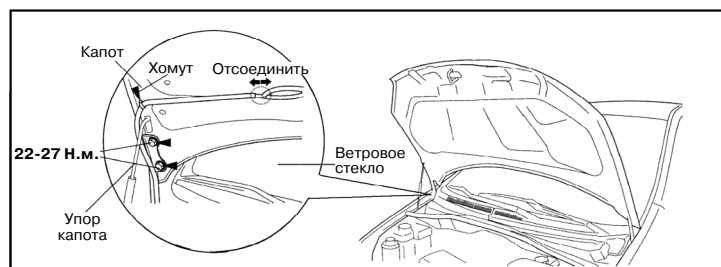
Рис. 2.1 – Элементы крепления капота.
