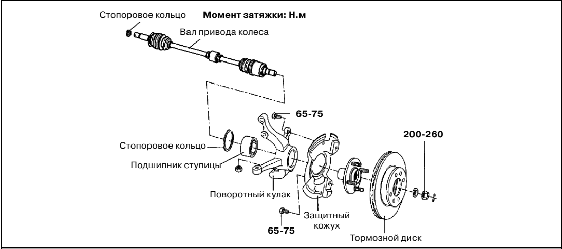
Рисунок 2.1 – Детали переднего привода
