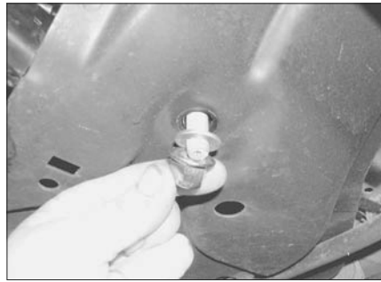
Рис. 19.7,а. Отверните гайки крепления рулевого механизма и снимите шайбы
