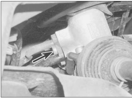
Рис. 19.5. Болт (указан стрелкой) прижимной планки питающей и возвратной трубок — модели с ГУР
