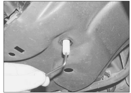
Рис. 19.7,б. ...затем выверните шпильки крепления...
