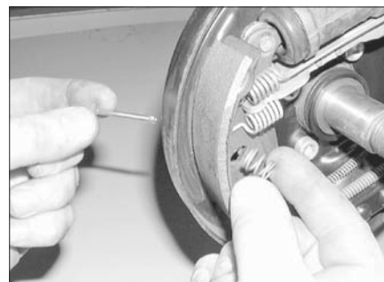
Рис. 6.6,в. ...снимите пружину и стойку
