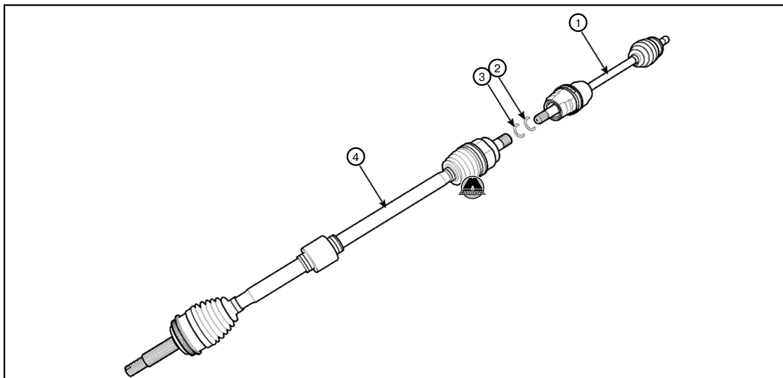
1. Приводной вал (левый) 2, 3. Стопорное кольцо 4. Приводной вал (правый)
