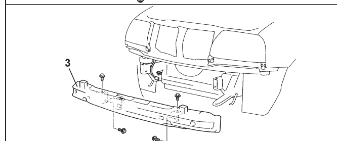
Передний бампер. 1 - решетка радиатора, 2 - передний бампер, 3 - усилитель переднего бампера.
