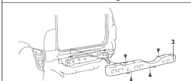
Задний бампер. 1 - накладка заднего бампера, 2 - задний бампер, 3 - усилитель заднего бампера.
