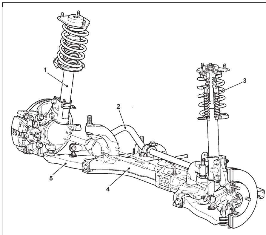
Общий вид передней подвески. 1 - стойка передней подвески в сборе, 2 - стабилизатор поперечной устойчивости, 3 - пружина, 4 - поперечная балка передней подвески, 5 - нижний рычаг.
