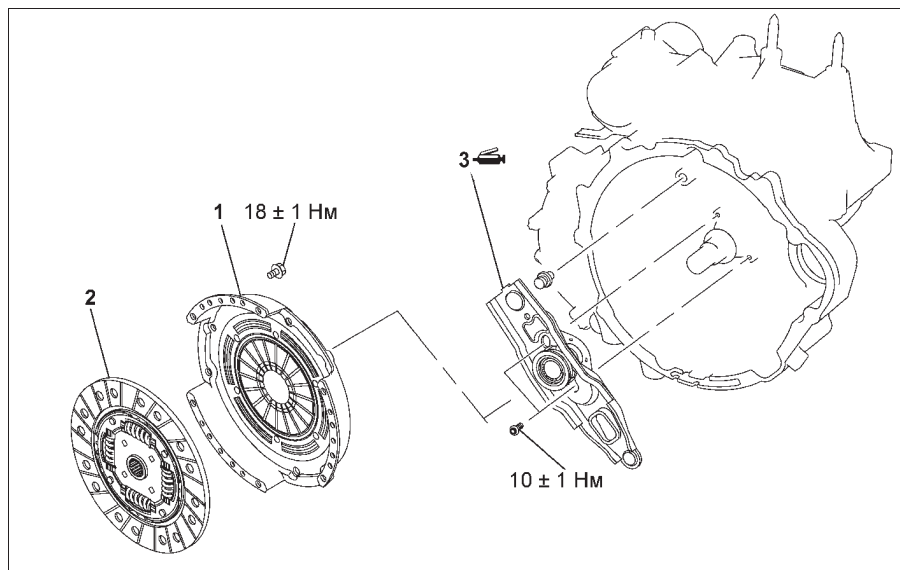
Снятие сцепления. 1 - кожух сцепления, 2 - ведомый диск сцепления, 3 - вилка выключения сцепления.
