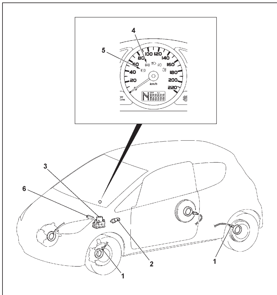
Компоненты системы ABS. 1 - датчик частоты вращения колеса, 2 - выключатель стоп-сигналов, 3 - гидравлический блок в сборе, 4 - индикатор "ABS", 5 - индикатор состояния тормозной системы и уровня тормозной жидкости, 6 - диагностический разъём.
