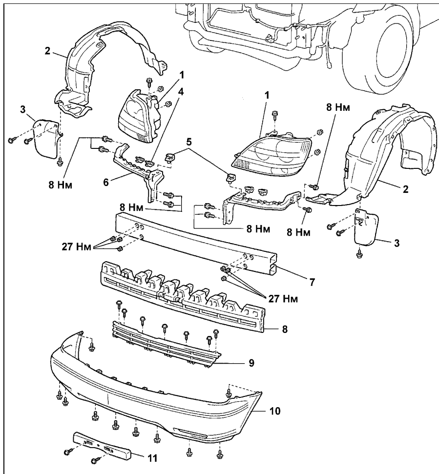
Передний бампер. 1 - фара, 2 - подкрылок, 3 - удлинительная подкладка, 4 - боковая опора бампера, 5 - кронштейн фары, 6 - накладка усилительная, 7 - усилитель бампера, 8 - гаситель энергии, 9 - решетка, 10 - накладка бампера, 11 - держатель номерного знака.
