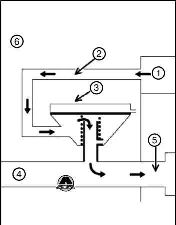
1. Крышка головки блока цилиндров 2. Шланг вентиляции картера 3. Клапан вентиляции картера 4. Отводящий воздухопровод воздушного фильтра 5. Турбокомпрессор 6. Атмосферное давление
