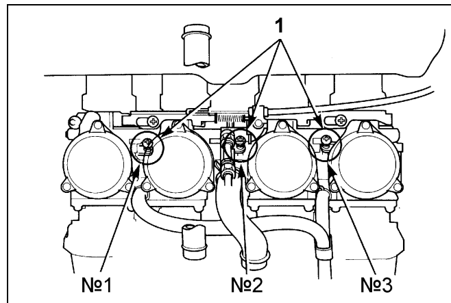
1 - регулировочные винты.
