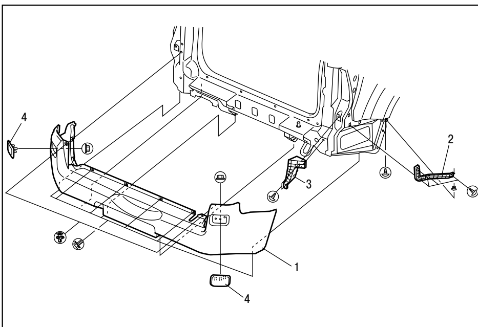
Задний бампер (3-х дверные модели). 1 – задний бампер, 2 – держатель №1 заднего бампера, 3 – держатель №2 заднего бампера, 4 – отражатель.
