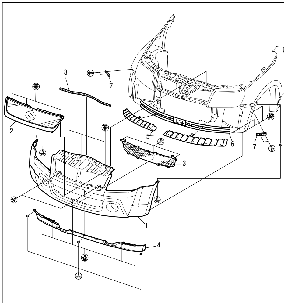
Передний бампер. 1 – передний бампер, 2 – решетка радиатора, 3 – сетка, 4 – отделка переднего бампера, 5 – энергопоглощающая вставка, 6 – установочная пластина, 7 – держатель переднего бампера, 8 – уплотнитель переднего бампера.
